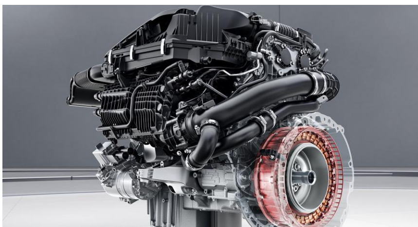
Tecnología EQ Boost: capaz de entregar hasta 22CV y 250Nm mediante el uso de alternador arrancador integrado de 48V
